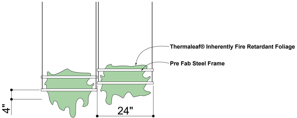
① ELEVATION 1
