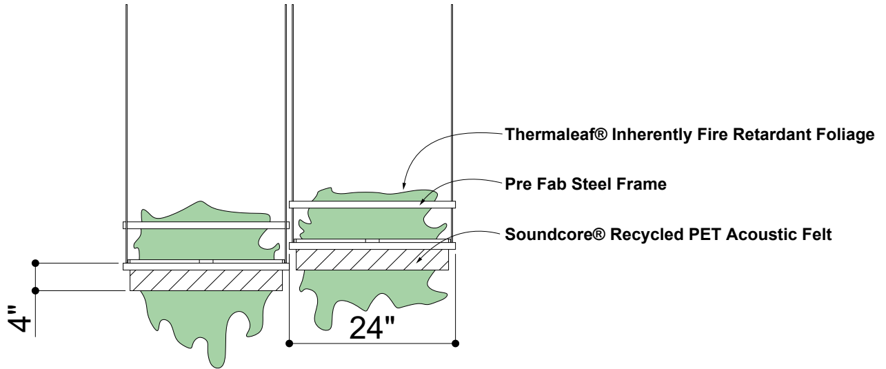
① ELEVATION 1
